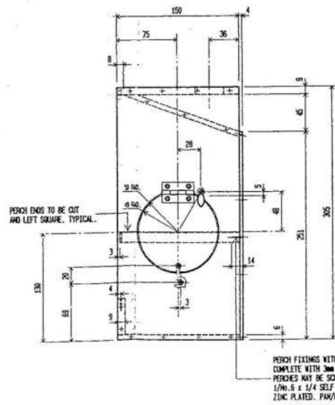
END ELEVATION
